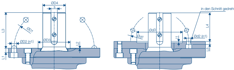
Anbausituation mit freiem Wellenende
