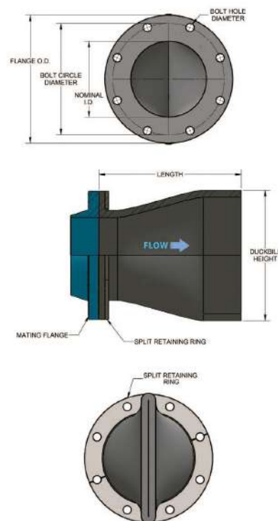
Detalhe Válvula Bico de Pato de Borracha Flangeada 710 ProFlex™
